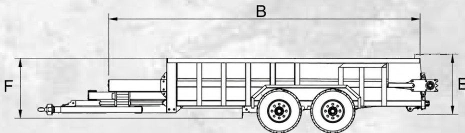
VISTA LATERAL
